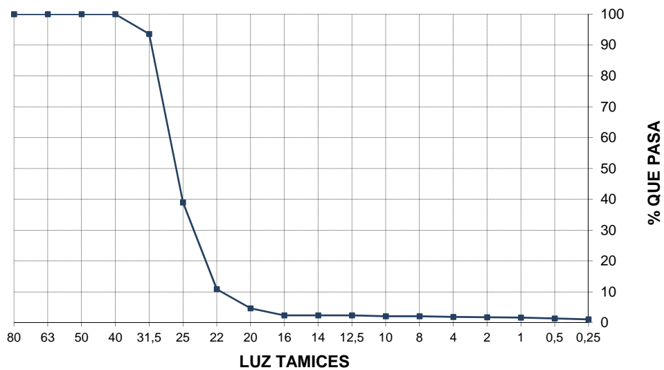
CURVA GRANULOMÉTRICA
