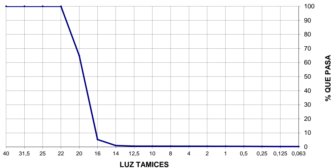
CURVA GRANULOMETRICA
