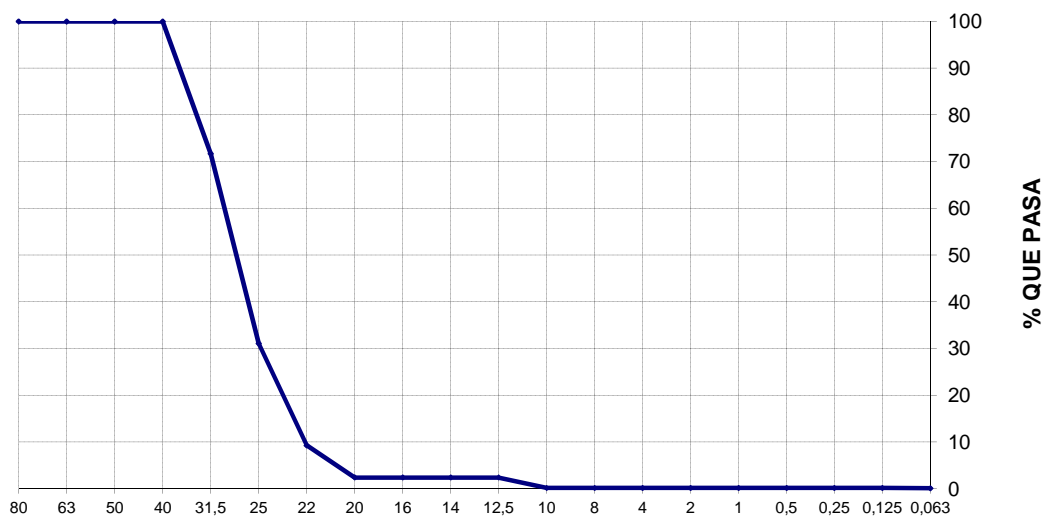
CURVA GRANULOMÉTRICA
