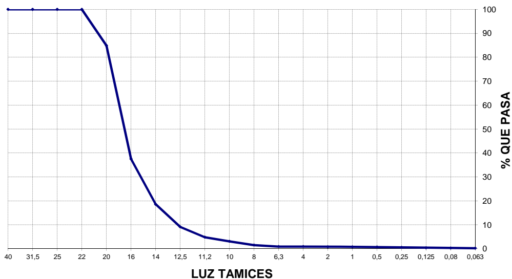
CURVA GRANULOMÉTRICA
