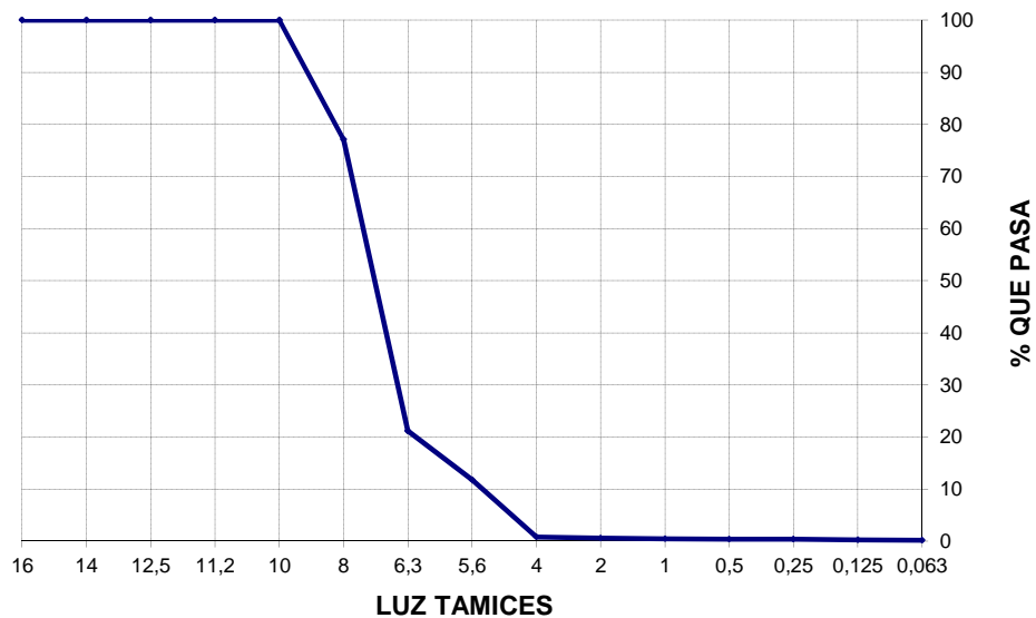
CURVA GRANULOMÉTRICA
