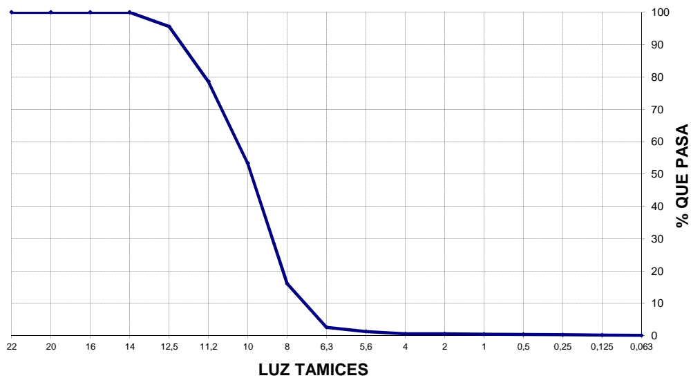
CURVA GRANULOMETRICA
