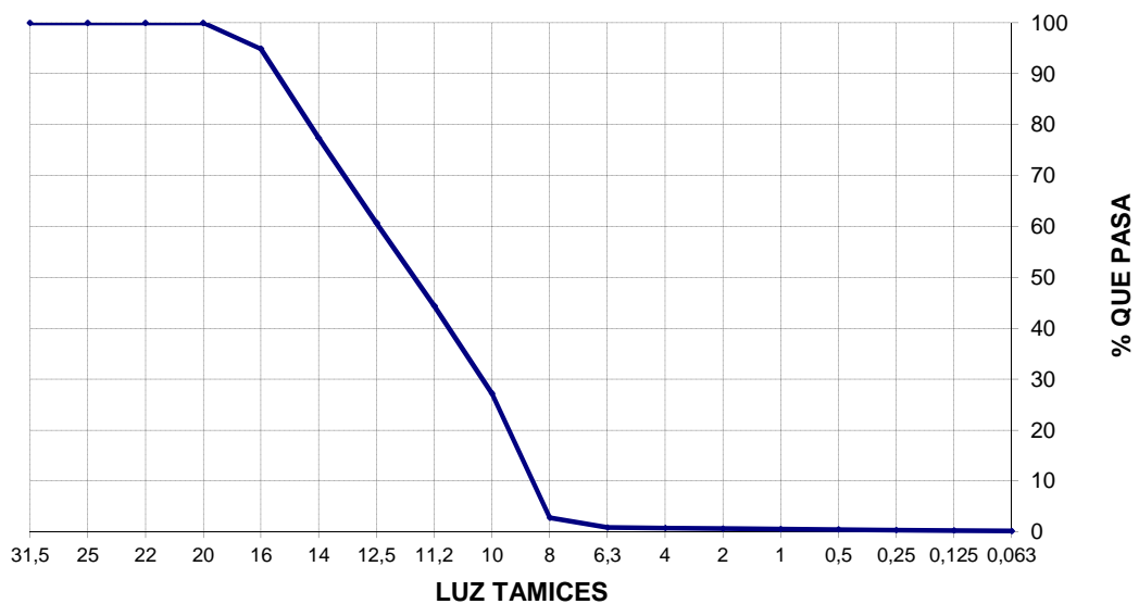
CURVA GRANULOMÈTRICA
